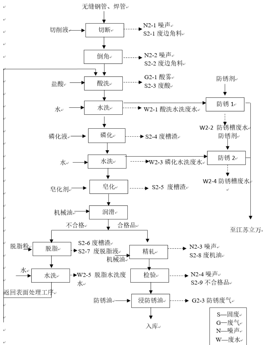
图 2.2-1 轴承钢管生产工艺流程图
